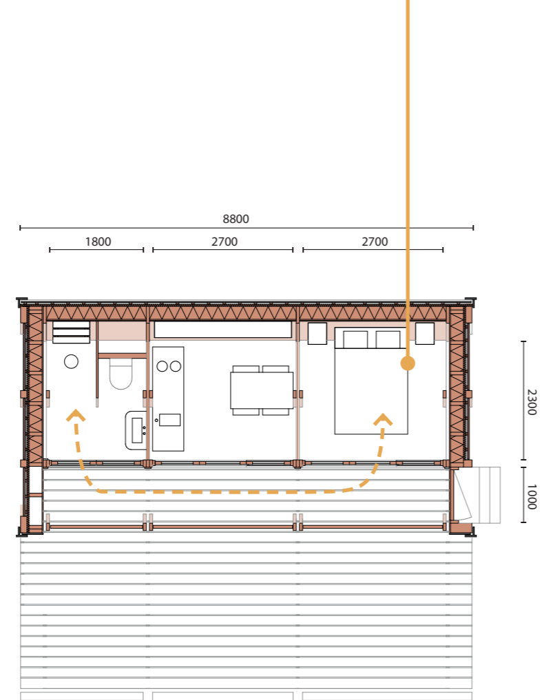
Slaapkamer - nacht
