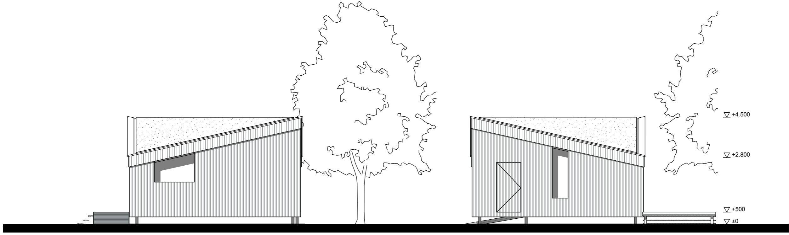
A-Locatie Gevelaanzicht 1:100 Rechtergevel
